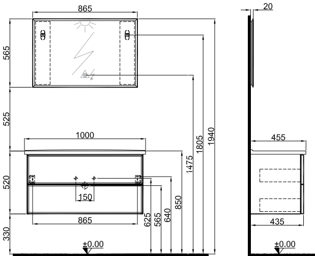
100 cm Lavabolu Dolap Ön ve Yan Görünüş
