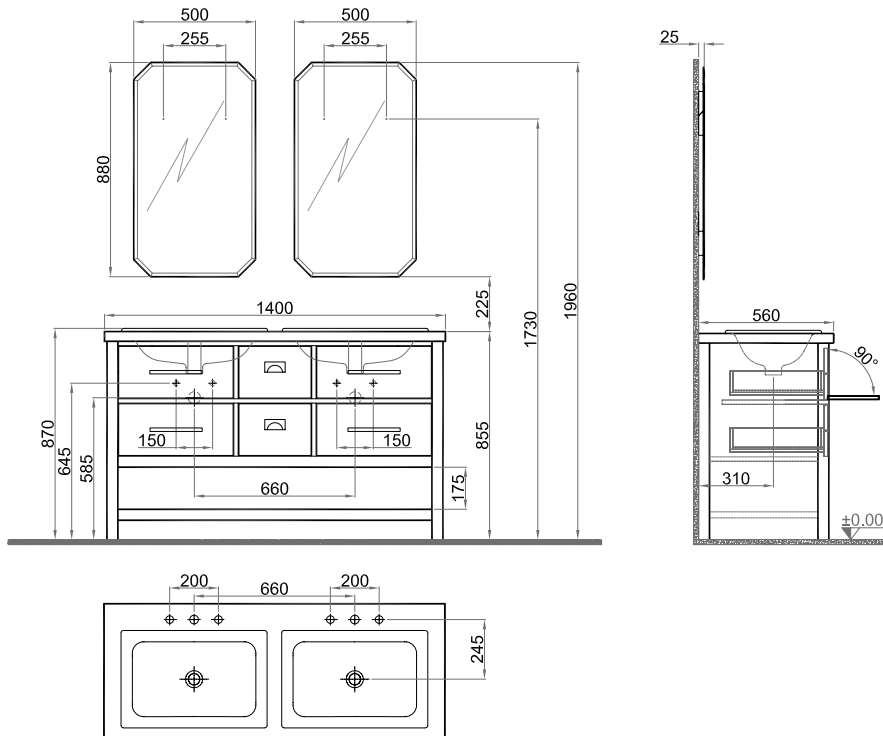
140 cm Lavabolu Dolap Ön ve Yan Görünüş
