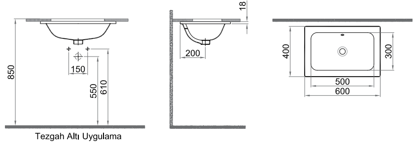
Tezgah Altı Uygulama
